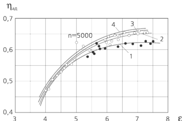
Рис. 3. Влияние конденсатосодержания газа на адиабатический КПД: 1 - d = 3 \text{ см}^3/\text{м}^3 ; 2 - d = 20 \text{ см}^3/\text{м}^3 ; 3 - d = 40 \text{ см}^3/\text{м}^3 ; 4 - d = 60 \text{ см}^3/\text{м}^3
