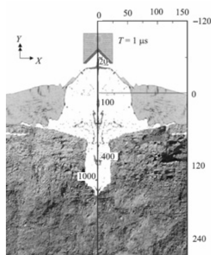
Рис. 2. Динамика развития взрывного взаимодействия кумулятивного заряда с разнопрочным массивом
