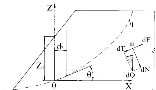
Рис. 2. Расчетная схема к определению положения экстремальной поверхности сдвига
