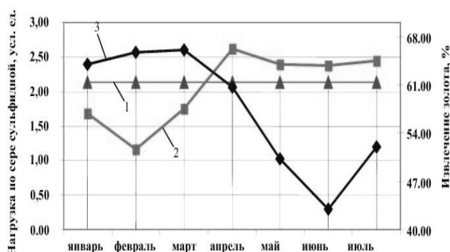
Рис. 1. Зависимость извлечения золота от нагрузки на схему биоокисления по сере сульфидной: 1- проектная нагрузка на схему биоокисления по сере сульфидной, т/сут; 2 - фактическая нагрузка на схему биоокисления по сере сульфидной, т/сут; 3 - извлечение золота, %
