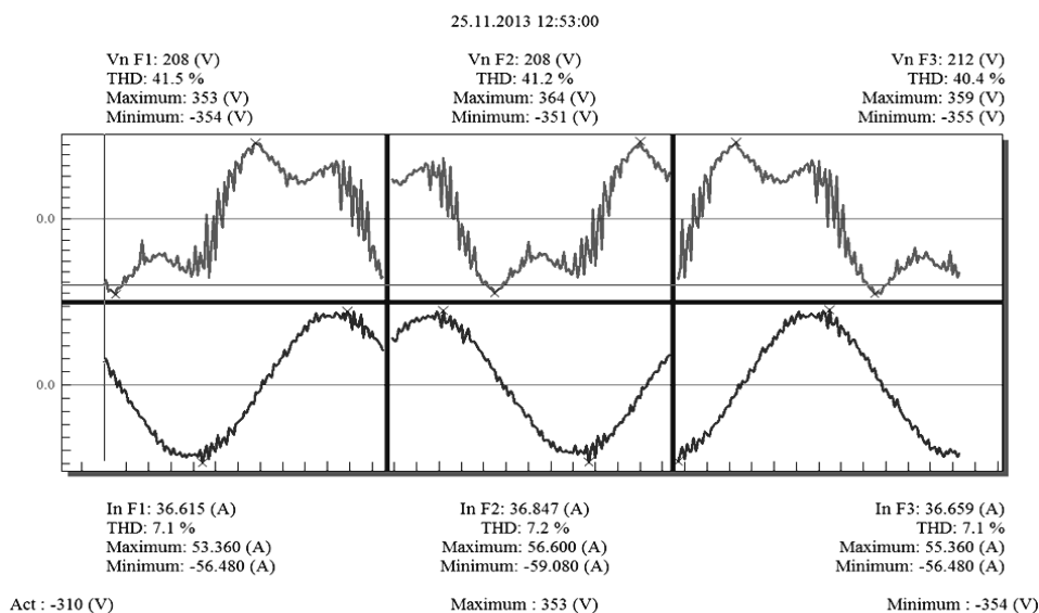
Рис. 4. Формы напряжения и тока каждой фазы в рабочем режиме питателя
