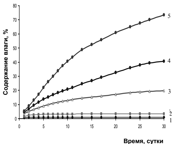
Рис. 5. Кинетика сорбции паров воды образцом 3 при относительных влажностях воздуха: 1-35%; 2-45%; 3-60%; 4-70% и 5-80%.
