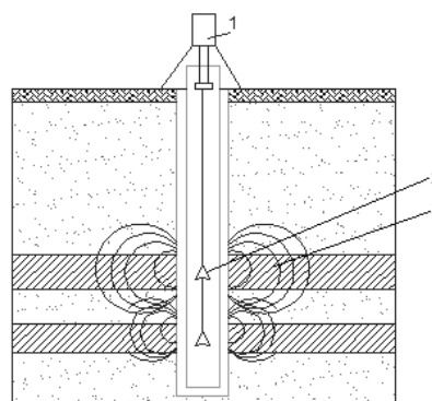
Рис. 12. Повышение проницаемости рудного массива гидроимпульсным воздействием: 1 - генератор волн; 2 - акустический отражатель; 3 - волны сжатия
