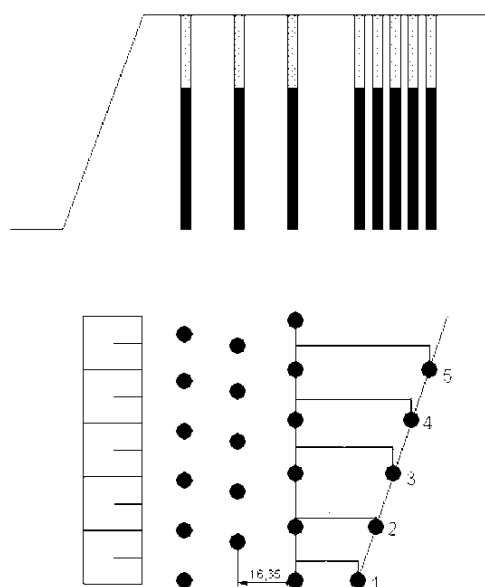
Рис. 2. Схема расположения скважинных зарядов ВВ в зоне ослабления прочности массива для установления расстояния между рядами: 1-5 – скважинные заряды ВВ
