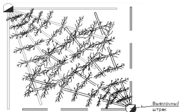
Рис. 10. Создание искусственной трещиноватости в скальных рудах поинтервальным гидроразрывом
