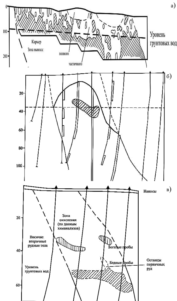
Рис. 2. Положение зоны окисления, уровня грунтовых вод и морфология рудных тел месторождений: а – Мурунтау; б – Мютенбай; в – Асаук;
