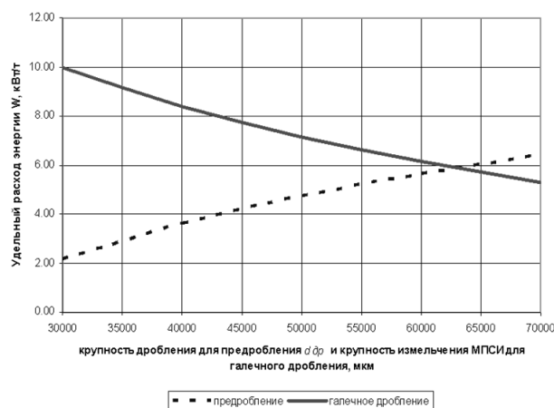
Рис. 4. Диаграмма удельного расхода электроэнергии для схем с предроблением и галечным дроблением для мягкой руды. Граничная крупность d_b -38000 мкм
