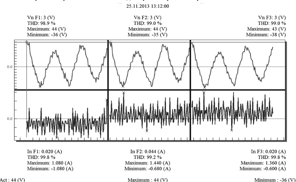
Рис. 5. Формы напряжения и тока каждой фазы в момент отключения питателя
