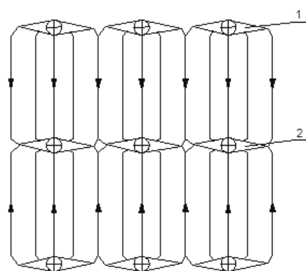
Рис. 8. Системы с линейными коллекторами в рядах технологических скважин: 1 - закачная скважина; 2 - откачная скважина
