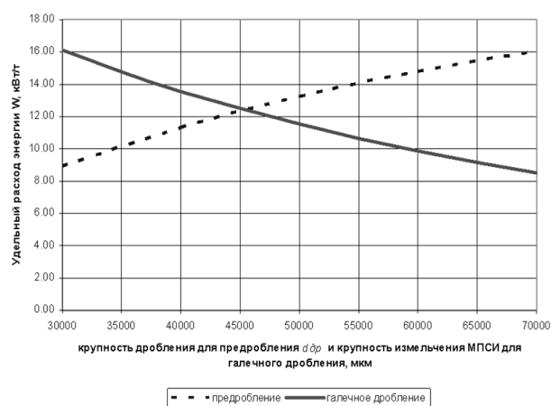
Рис. 5. Диаграмма удельного расхода электроэнергии для схем с предроблением и галечным дроблением для твердой руды. Граничная крупность d_b -20000 мкм
