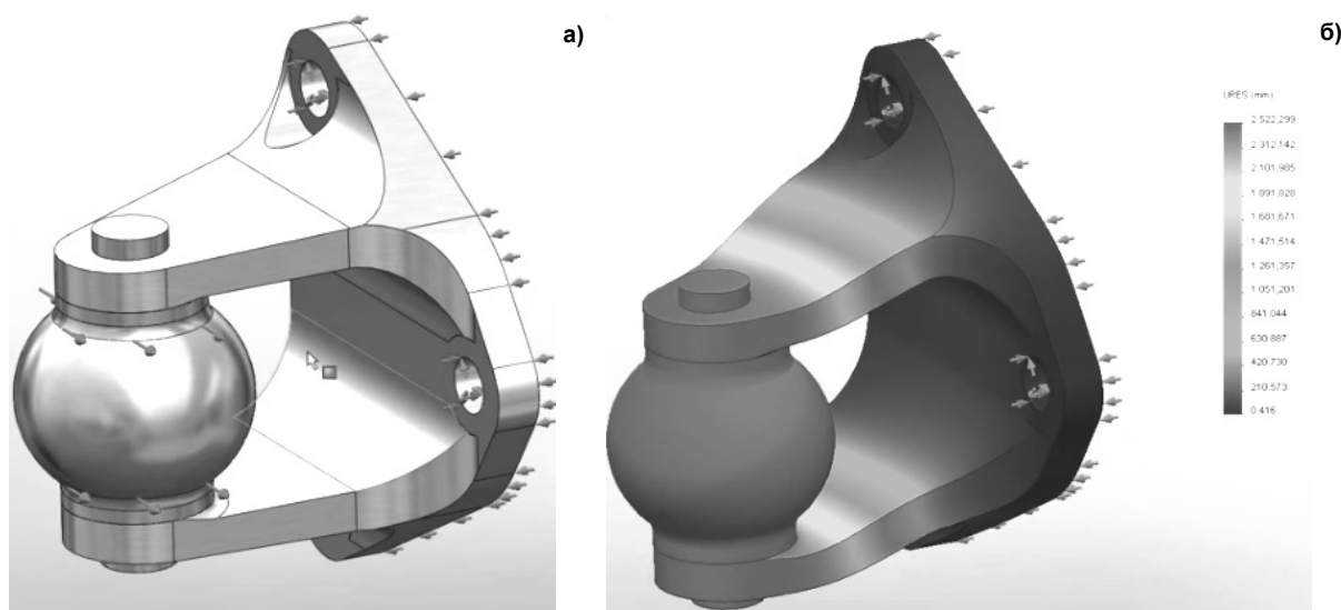
1 - расм. Материал ва металлларнинг зичлигини ҳамда ички кучланишларни таъсири кўриниши: а) йиғилган ролик детали; б) ролик деталини маҳкамлаш ва таъсир этувчи куч йўналишларини ўрнатиб хавфли кесимини топиш
