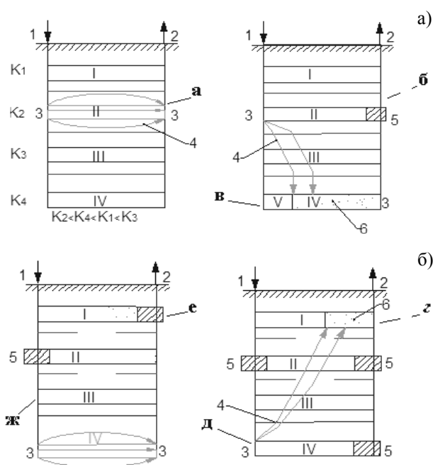
Рис. 6. Способ обработки многопластового месторождения: 1 - закачные скважины; 2 - откачные скважины; 3 - фильтр; 4 - линии тока; 5 - закольматированная зона; 6 - частично закисленная зона
