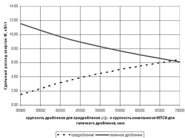
Рис. 6. Диаграмма удельного расхода электроэнергии для схем с предроблением и галечным дроблением для рудника N. Граничная крупность d_b -45000 мкм
