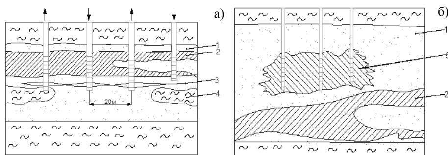
Рис. 1. Системы ПВ с локализацией растворов: а - гидроразрывными экранами; б - колюматационными завесами (1-рудный горизонт; 2-рудное тело; 3-противофильтрационный экран; 4-водоупор; 5-колюматационная завеса)
