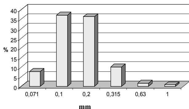
Рис. 2. Гранулометрический состав кварцевого песка Яккабагского месторождения
