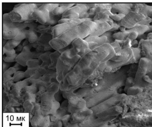
Рис. 12. Фракталы ртутистого золота: а) слои роста нанометровой ширины; б) с элементом микропористой текстуры [10]
