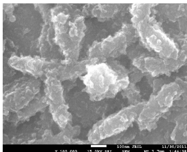
Рис. 14. Сложные выделения «нового» золота удлинённой формы [5]
