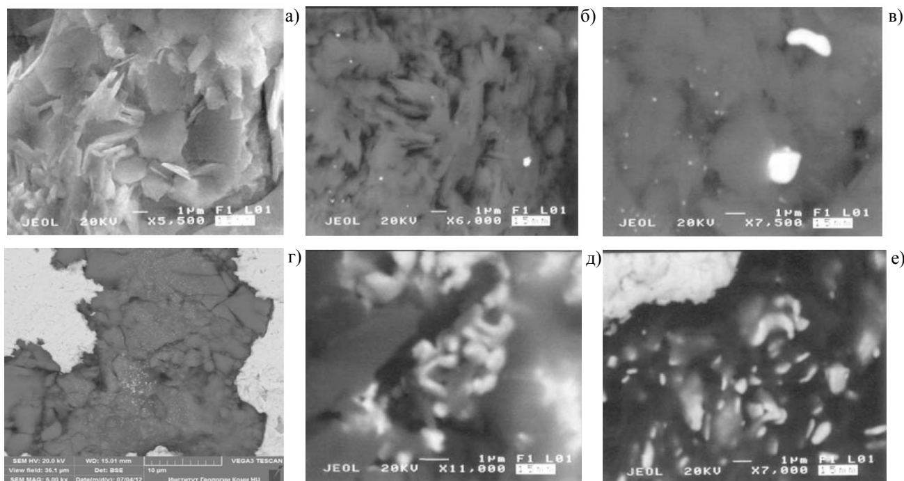
Рис. 6. Тонкодисперсные минералы на поверхности золотин [4]: а, б - слюды и гидрослюды; в - гидроксиды железа; г - е - тонкодисперсная окисно-алюмосиликатная масса (темное); б-е - наночастицы золота (белое). Золотины из россыпей р. Кыввож (а-в), Естошор (г), руч. Ветвистый (д), руч. Кыяншор (е). РЭМ-изображения во вторичных (а, г) и упругоотраженных (б, в, д, е) электронах
