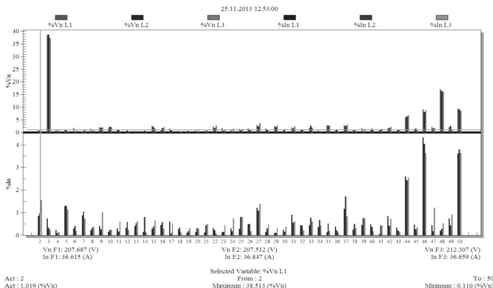
Рис. 2. Мгновенные значения гармонического состава напряжения и тока до 50 гармоник
