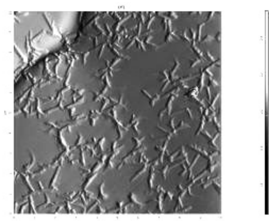
Рис. 16. Атомно-силовое изображение поверхности агломерированного золота [16]
