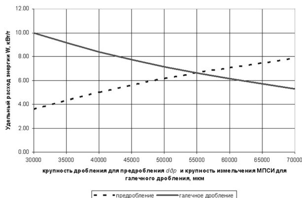
Рис. 3. Диаграмма удельного расхода электроэнергии для схем с преддроблением и галечным дроблением для средней руды. Граничная крупность d_b -29000 мкм
