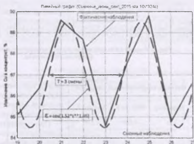
Рис. 2. Оценка гармонической составляющей случайной функции \epsilon = f(t) .
