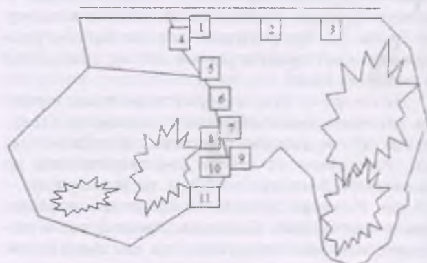
Рис. 5. Предлагаемая схема переработки сбросовых пульп золотоизвлекательных фабрик.
