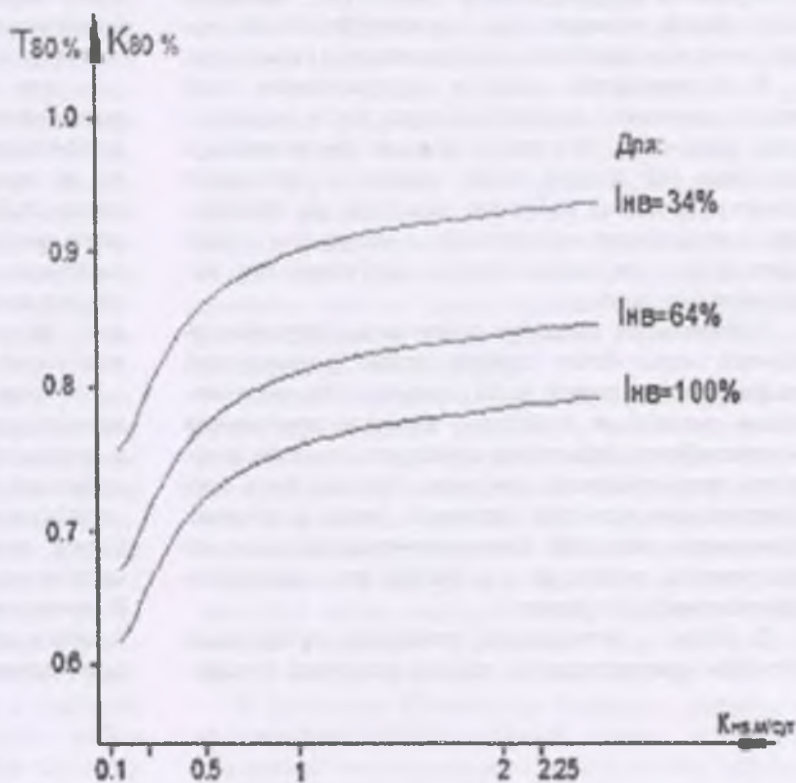
Рис. 6. Зависимость времени отработки ( T_{80\%} ) единичной ГДЯ и расхода реагента ( K_{80\%} ) от проницаемости ( K_{ис} ) и площади ( I_{ис} ) искусственного водоупора.
