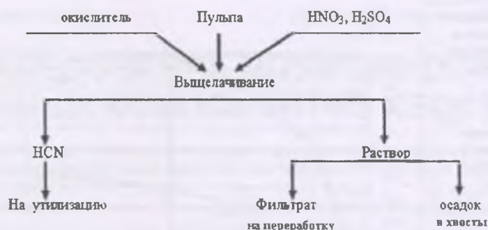
Рис. 5. Предлагаемая схема переработки сбросовых пульп золотоизвлекательных фабрик.
