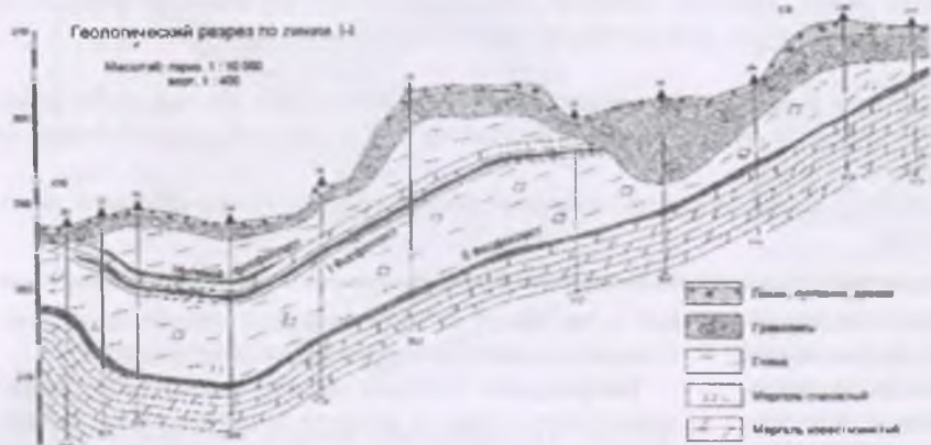
Рис. 1. Горно-геологический разрез месторождения Джерой-Сардара.
