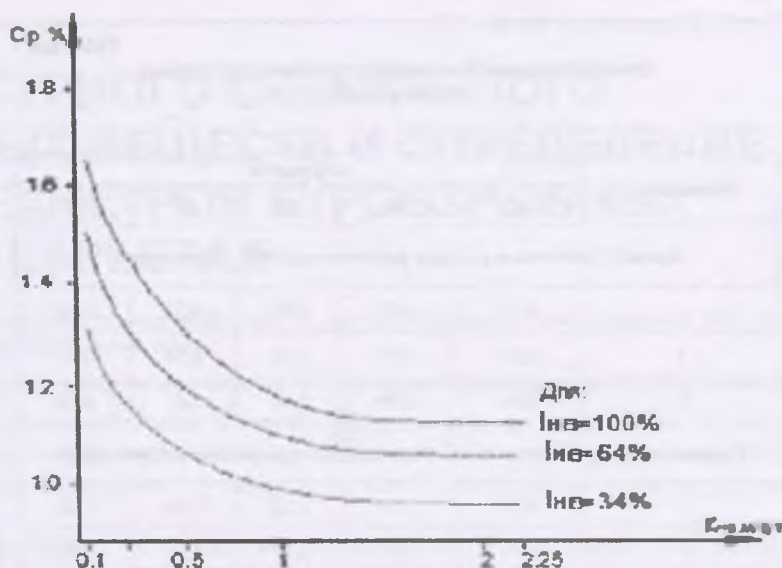
Рис. 5. Зависимость среднего содержания полезного компонента ( C_{ср 80\%} ) от проницаемости ( K_{ис} ) и площади ( I_{ис} ) искусственного водоупора.
