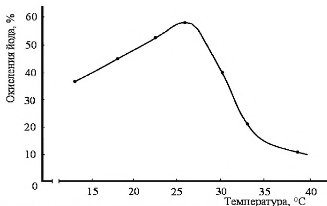
Рис.1. Зависимость температуры системы на процесс окисления йодида иона (рН=3, окислитель NaClO)
