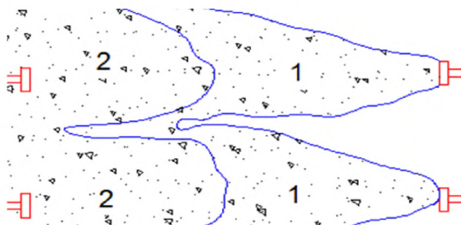
Рис. 3. Горизонтальный разрез коагуляции: 1-Зона коагуляции; 2-Зона интенсивной коагуляции
