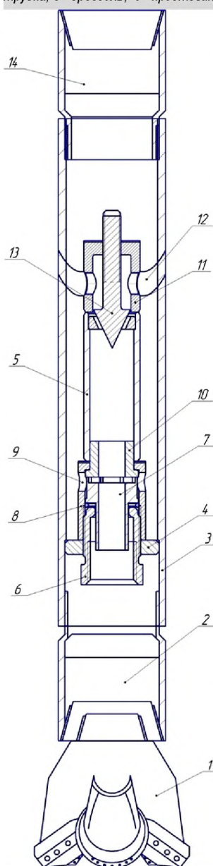
Рис.5. Буровой снаряд включающий в себя вихревую трубу для бурения с очисткой забоя воздухом. 1-шарошечное долото; 2-переходник; 3-наружная трубка; 4-перемычка (шайба); 5-вихревая труба; 6-гайка; 7-генератор холодной фракции на холодном выходе; 8-корпус; 9-входное отверстие; 10-шайба; 11-корпус дросселя на горячем выходе; 12-тангенциальное отверстие для выхода горячего воздуха; 13-дроссель на горячем выходе; 14-верхний переходник
