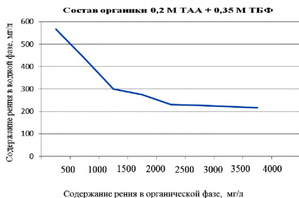
Рис.2. Изотерма экстракции рения при составе органики 0,2М ТАА+ 0,35М ТБФ
