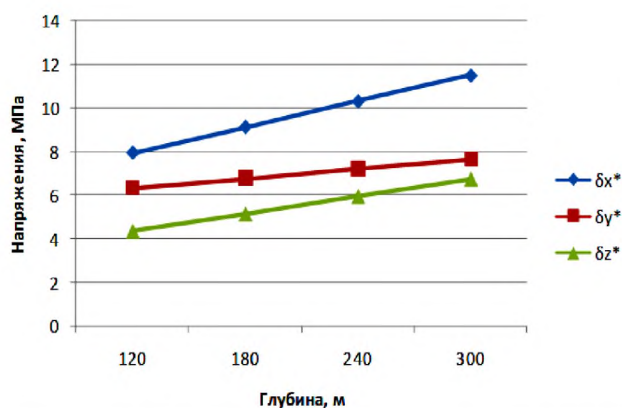
Рис.1. График зависимости напряжений в горном массиве от глубины ведения горных работ
