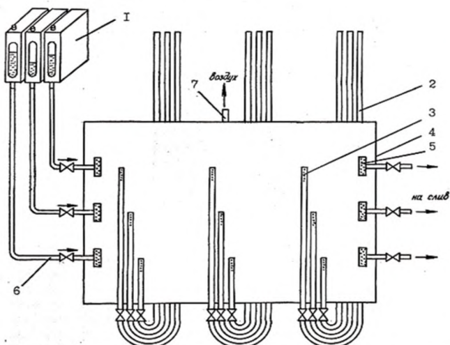
Рис.1. Фильтрационный лоток: 1-Напорные бочки; 2-Пьезометрические трубки; 3-Пьезометрические скважины; 4-Корпус стенда; 5-Фильтры скважины; 6-Соединительные шланги; 7-Отверстие для дегазации
