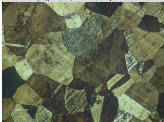
Рис.4. Микрофотография стали 110Г13Л после закалки, T_{зак} = 1100^\circ C (x 100)
