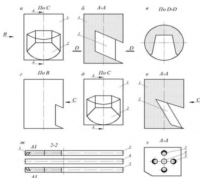
Рис.2. Схемы асимметрических цилиндрических кумулятивно-канальных зарядов: 1 – патрон прессованного аммонита (литого тротила или рассыпного ВВ); 2 – кумулятивная выемка; 3 – врубные шпур; 4 – сорентированная выемка в сторону компенсационного шпура или обнаженного пространства
