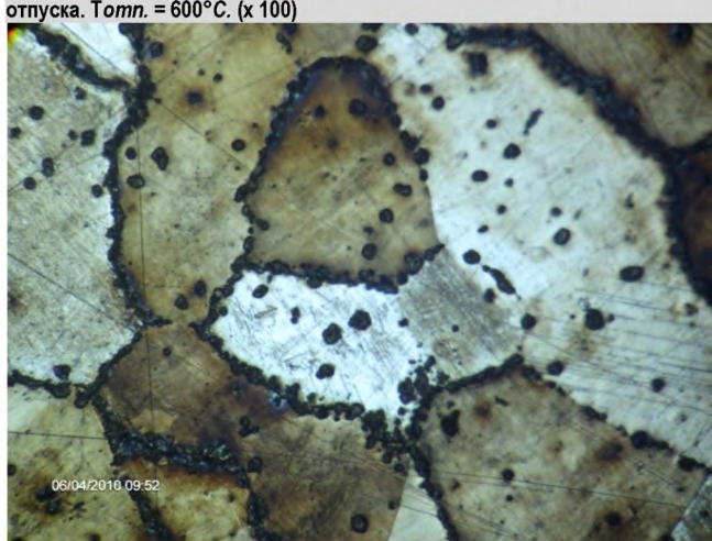
Рис 8. Рост зерна аустенита и появление карбидов в теле и по границам зерен аустенита стали 110Г13Л. (x 100)
