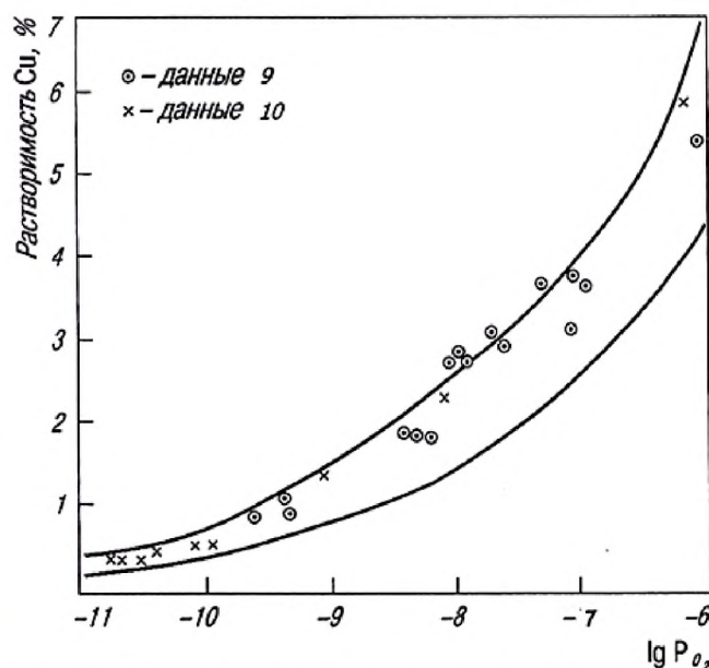
Рис. 3. Влияние парциального давления кислорода на растворимость меди в шлаках
