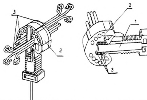
Рис.3. Схема подсоединения волноводов устройств в монтажные соединители: 1 – капсюль-детонатор с замедлением; 2 – монтажный соединитель; 3 – волноводы инициирующих устройств
