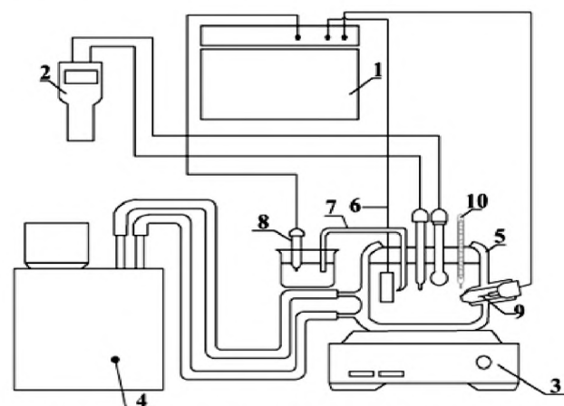
Рис.2. Схема лабораторной установки электроокислации MoK в растворе 10% NaCl: 1 - потенциостат ПИ-50-1, 2 - pH-метр, 3 - мешалка, 4 - термостат, 5 - ячейка, 6 - анод, 7 - капилляр Лугина, 8 - х.с. электрод, 9-катод, 10 - термометр
