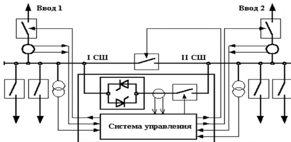
Рис.1. Схема быстродействующего автоматического ввода резерва
