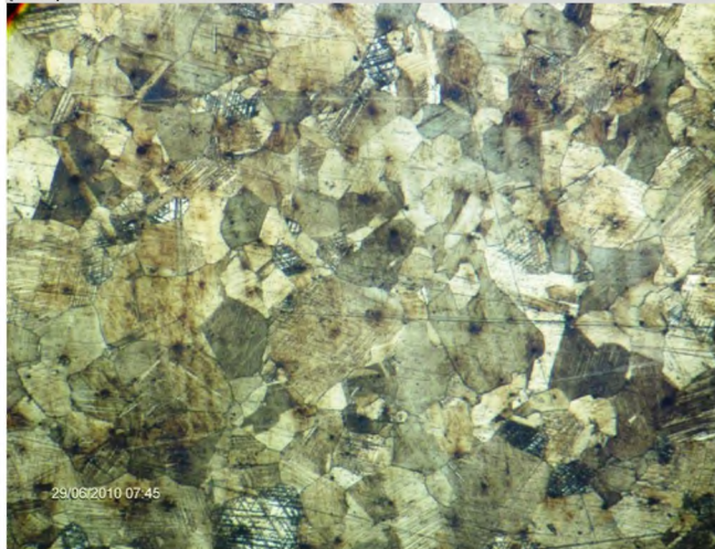
Рис.7. Мелкие зерна аустенита стали 110Г13Л после предварительного отпуска. T_{отп.} = 600^\circ C . (x 100)
