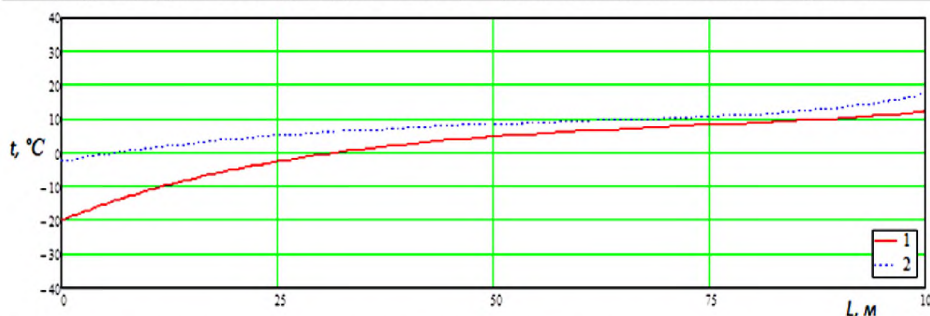
Рис.3. График распределения температуры t в бурильных трубах (1) и кольцевом канале (2) по глубине скважины
