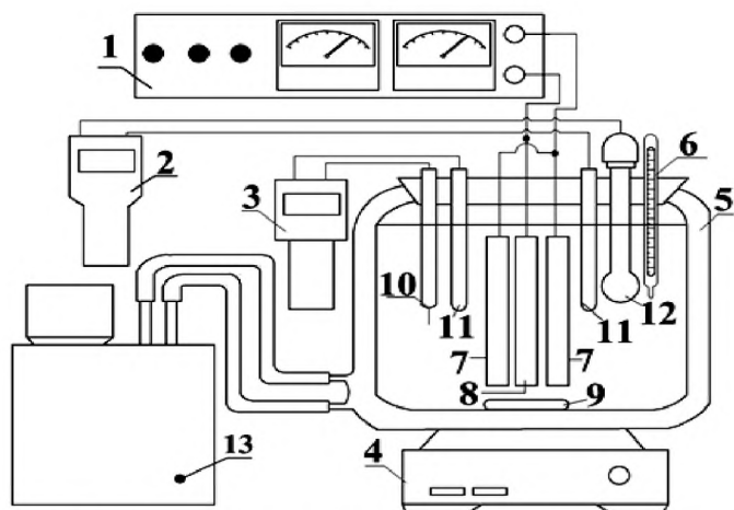
Рис.1. Схема пилотной установки электроокислации MoK в растворе 10% NaCl: 1-источник тока, 2 - pH метр, 3 - ЭВ-74, 4 - мешалка, 5-электролизер, 6-термометр; 7,8- электроды 9 – магнит; 11,13 – х.с. электрод сравнения, 12 – стеклянный электрод, 14-термостат
