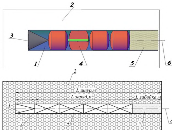
Рис.4. Конструкция шпуровых зарядов с кумулятивным эффектом: 1 – шпур; 2 – массив горных пород; 3 – конус из металлической облицовки; 4 – заряд ВВ; 5 – забойка; 6 – источник инициирования
