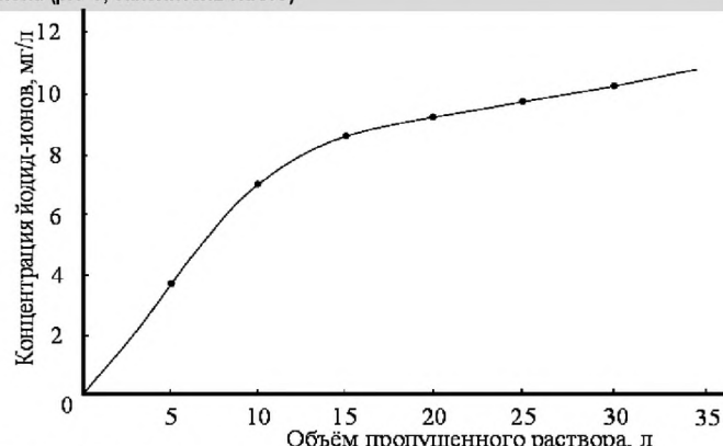
Рис.2. Выходная кривая сорбции йода из естественных растворов с C_i = 10 \text{ мг/л}
