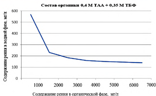
Рис.4. Изотерма экстракции рения при составе органики 0,4М ТАА + 0,35М ТБФ
