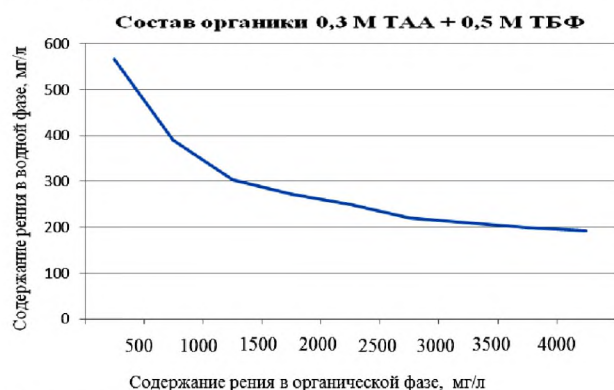
Рис.3. Изотерма экстракции рения при составе органики 0,3М ТАА+ 0,5М ТБФ
