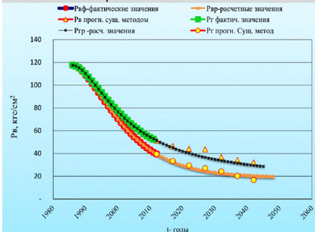
Рис. 5. Зависимость средневзвешенного давления воды P_v и газа P_g в кгс/см^2 от времени t
