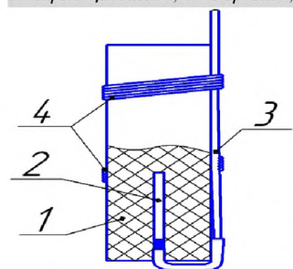
Рис.2. Схема инициирования эмульсионного патрона ВВ: 1 – патрон ВВ; 2 – капсюль-детонатор; 3 – волновод устройства; 4 – шланг, лента клейкая
