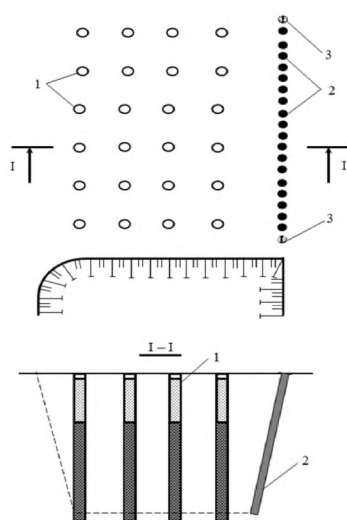
Рис.1. Схема расположения экранирующих контурных скважин: 1 – взрывные скважины; 2 – экранирующие контурные скважины; 3 – боковые скважины с установленными металлическими дугообразными пластинами
