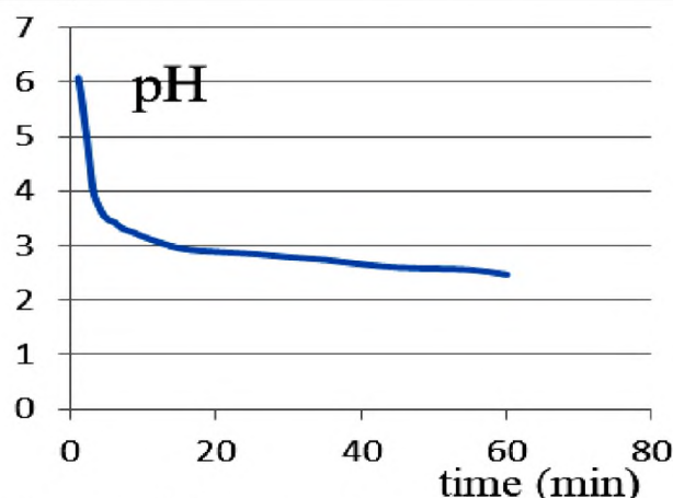
Рис.3. Изменение pH в 2-камерном мембранном электролизере, гальваностатический режим I=2,45 \text{ mA} , 75 \text{ cm}^3
