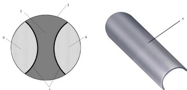
Рис. 2. Конструкция боковой экранирующей контурной скважины с металлическими пластинами дугообразной формы: 3 – боковая экранирующая контурная скважина; 4 – металлическая дугообразная пластина; 5 – невзрывчатая разрушающая смесь; 6 – буровая мелочь
