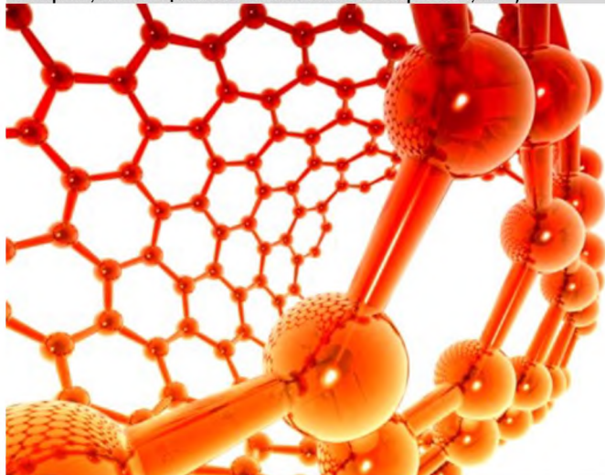
Рис. 3. Золотой фуллерен
