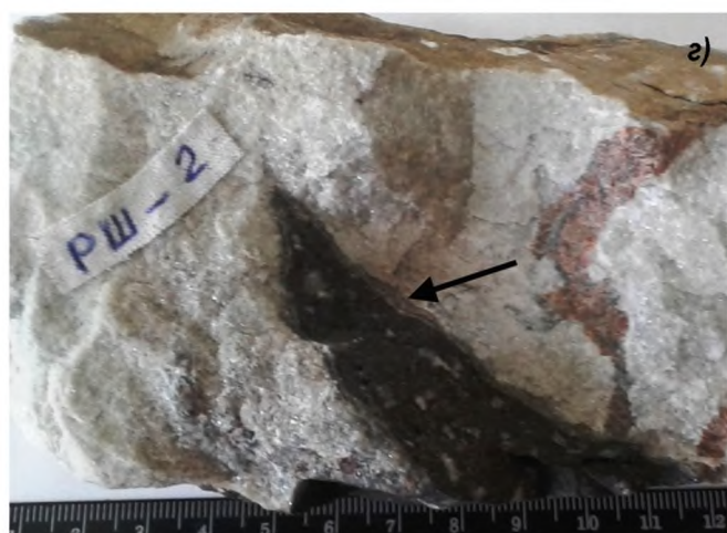
Рис.2. Фрагменты взаимоотношения даек с вмещающими породами на полосе Койташ-Угат: а- схема взаимоотношения гранодиоритов, даек диоритовых порфиров и сульфидно-редкометалльных руд полосы Койташ-Угат, горизонт 700 м [Хамрабаев и др., 1993]. 1-диоритовый порфирит (Т 1 ), 2-гранодиорит (Р 1 ), 3-мраморизованный известняк (С 2 ), 4-роговик (С 2 ), 5-скарны и скарнированные породы убогосульфидные, 6-скарново-сульфидные (пирротин-халькопирит-пирит) залежи, 7-ксенолиты руд в диоритовом порфирите; б- контакт гранодиорита Койташского интрузива с дайкой лампрофира, в- образования сульфидного прожилка на контакте; г- прорывание лампрофировой дайки на мраморизованные известняки, где скарнируется (тонкая полоса указан стрелкой, шахта «Главная»); д- контакт лампрофировой дайки с терригенно-карбонатными породами (шахта «Главная»)
