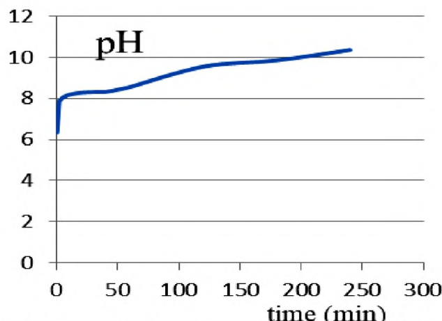
Рис.4. Изменение pH в 1-камерном электролизере, гальваностатический режим I=109,9 \text{ mA} , 75 \text{ cm}^3
