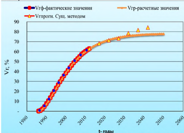
Рис. 4. Зависимость суммарного количества отобранного газа от начальных запасов V_{гг} в % от времени t
