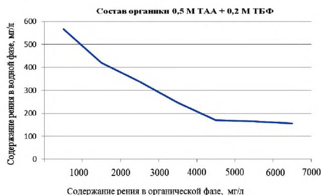
Рис.5. Изотерма экстракции рения при составе органики 0,5М ТАА + 0,2М ТБФ
