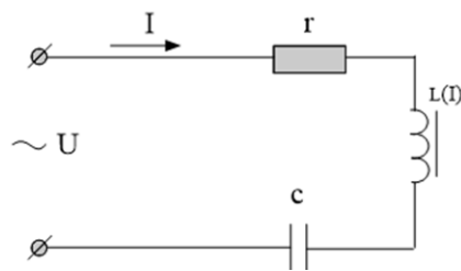
1-rasm. Rostlanmaydigan nochiziqli induktivlik va chiziqli elektr zanjirlari
