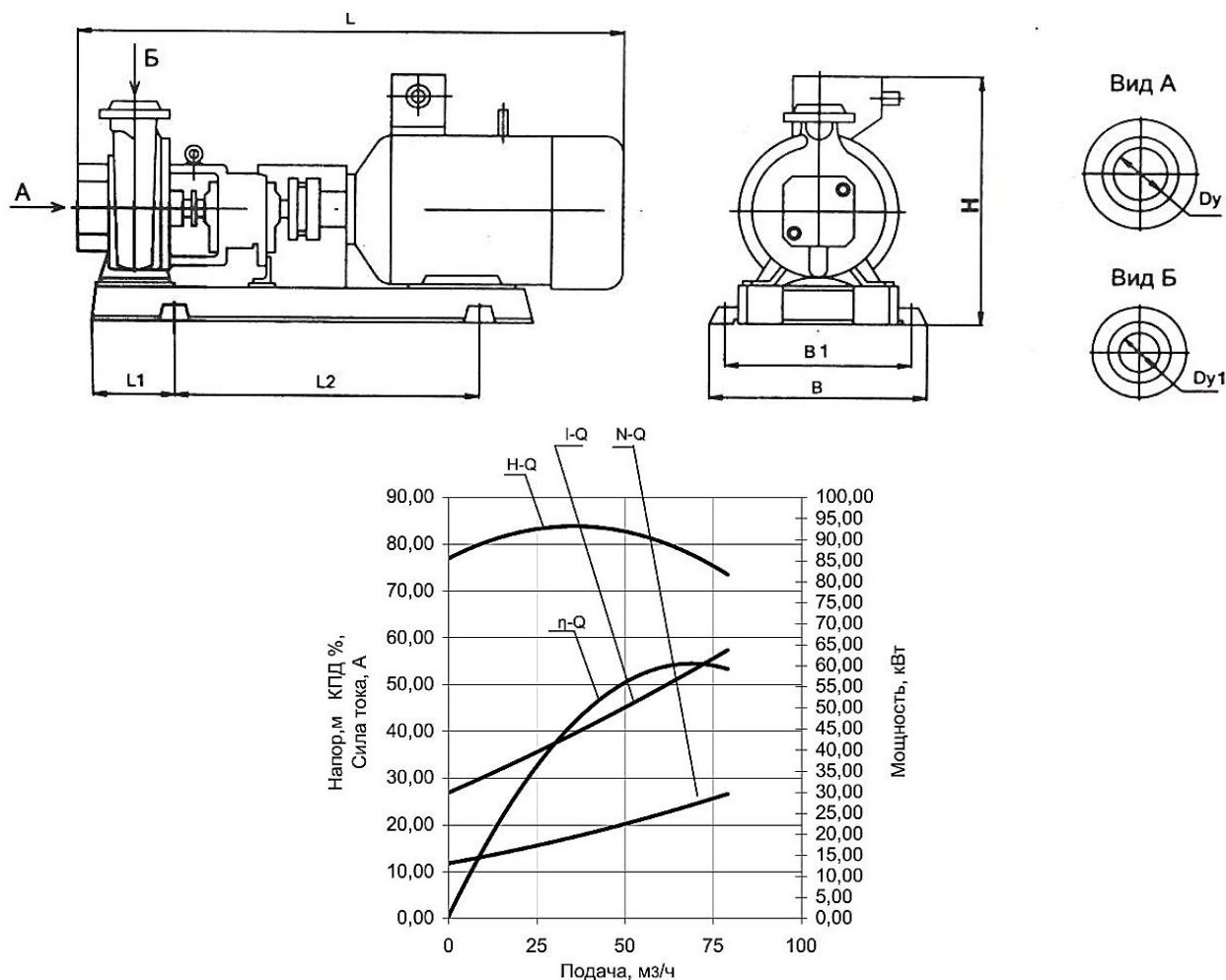
Рис. 5. Схема работы и чертёж насоса К80-50-250: H-Q – напор H (м) в зависимости от подачи Q (м³/ч); η-Q – КПД η (%) в зависимости от Q (м³/ч); I-Q – сила тока двигателя III (А) в зависимости от Q (м³/ч); N-Q – потребляемая мощность N (кВт) в зависимости от Q (м³/ч)
