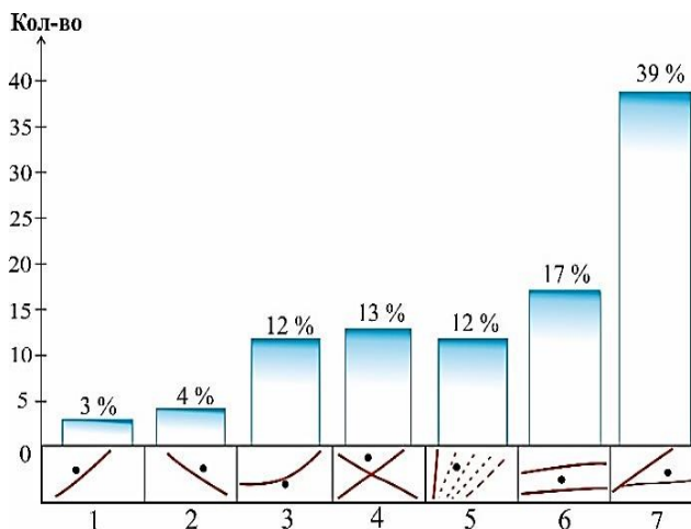
Рис. 2. Распределение золоторудных проявлений Бельтау по структурным позициям: 1 – зона северо-восточного разлома; 2 – зона северо-западного разлома; 3 – зона искривления разлома; 4 – зона пересечения разломов; 5 – зона скальвания; 6 – зона субпараллельных разломов; 7 – зона клиновидной структуры
