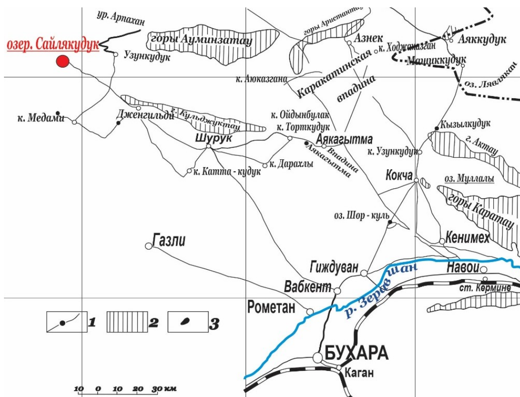
Рис. 1. Обозначенная карта распространения современного солёного озера Сайлякдук в Центральных Кызылкумах: 1 – маршруты и точки наблюдений в зонах засоления; 2 – выходы пород палеозойского возраста; 3 – крупнейшие солёные озёра и месторождения (указаны схематично)
