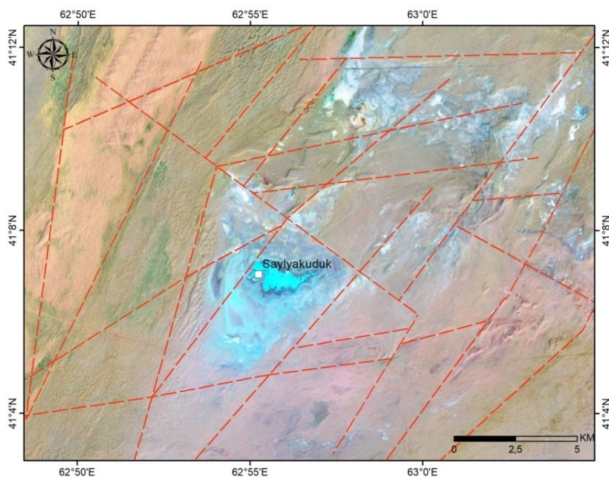
Рис. 2. Космоструктурная схема участка озера Сайлякүдүк (масштаба 1:100 000)
